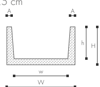
NOMA® BEAM Trave 15x15
